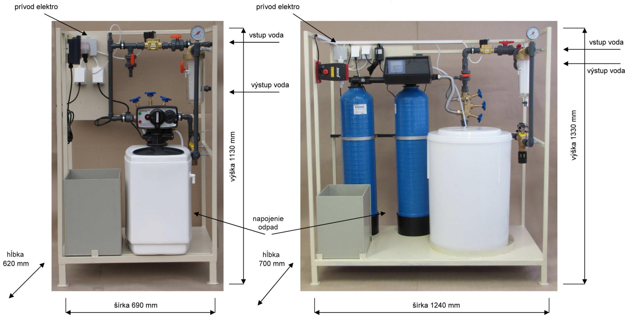
BUV s kabinetovým zmäkčovacím filtrom
