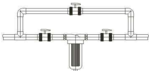
štandardná inštalácia s obtokom
