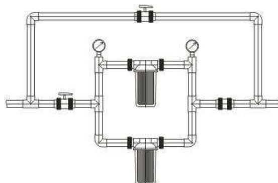
paralelná inštalácia pre vyšší výkon / čistenie za prevádzky
